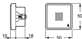
IHC CONTROL® Klimastyring Fugt- og temperatur-sensor LK FUGA
