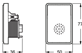
IHC CONTROL® Alarm lydgiver Intern LK FUGA
